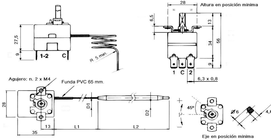
Termostato
