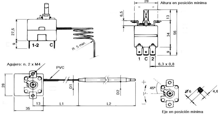
Termostato
