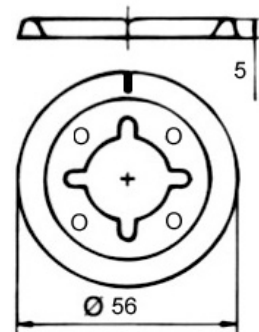
Embellecedor cromado
