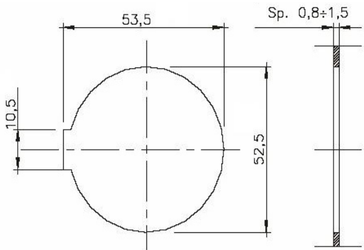
Dimensiones Panel
